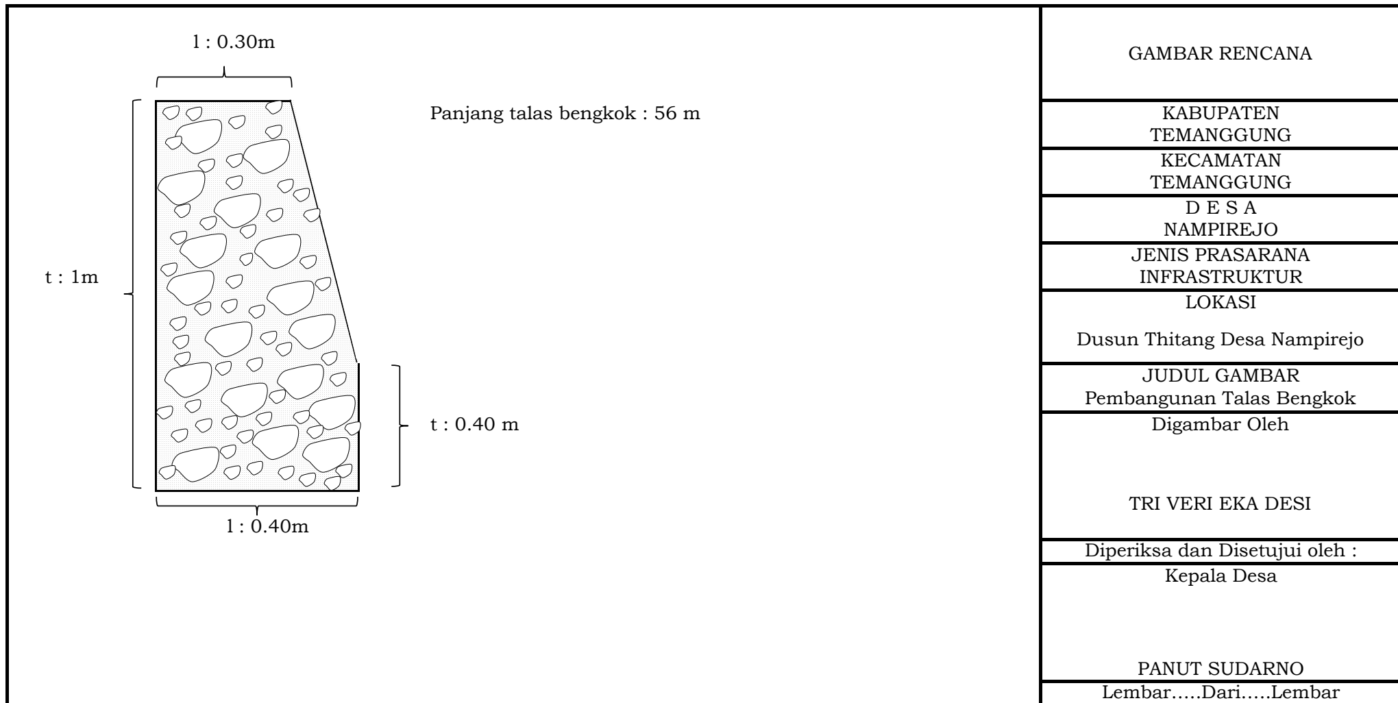
GAMBAR RENCANA PRASARANA
